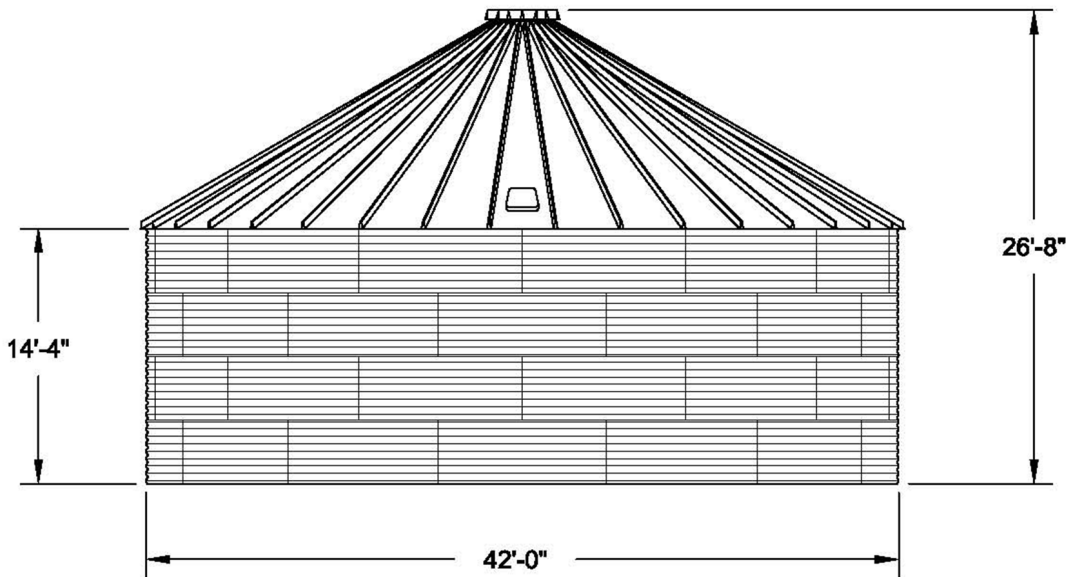
ELEVATION
